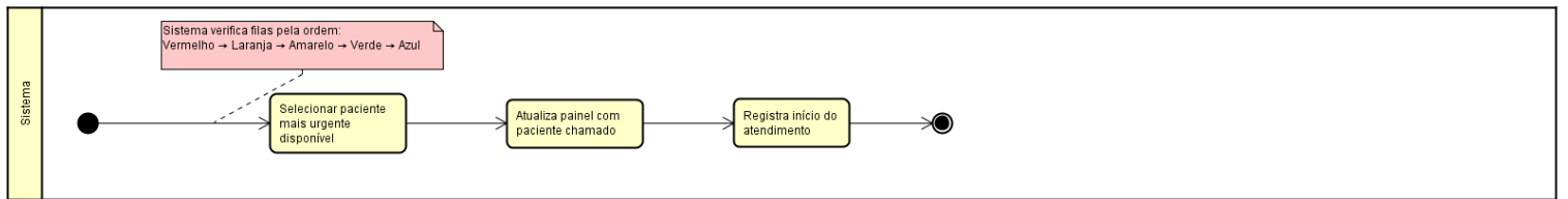
act PN - Chamada para Atendimento / Painel (Nível 1)
